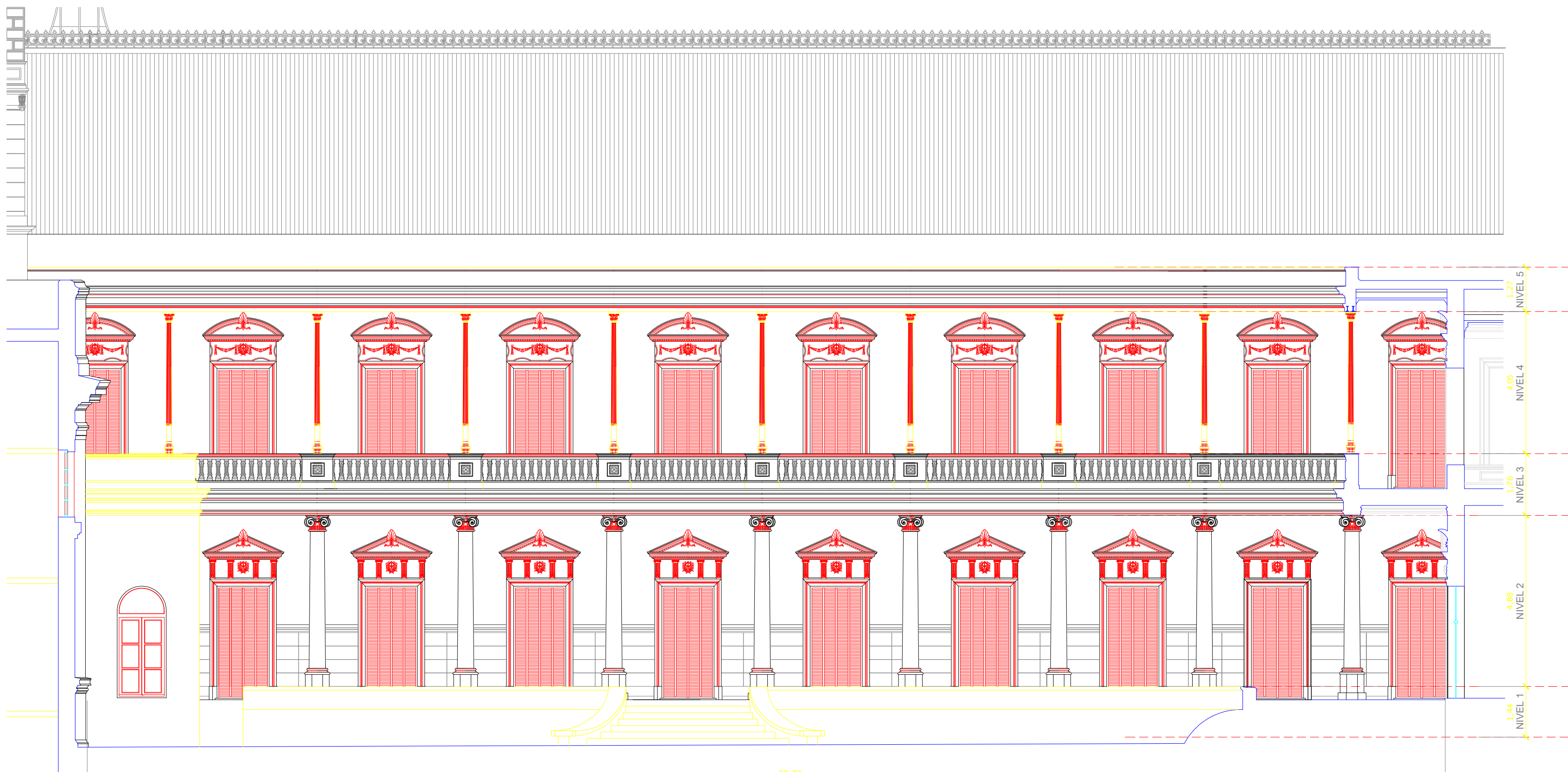
PATIO SUR - FACHADA OESTE ESC. 1:50
