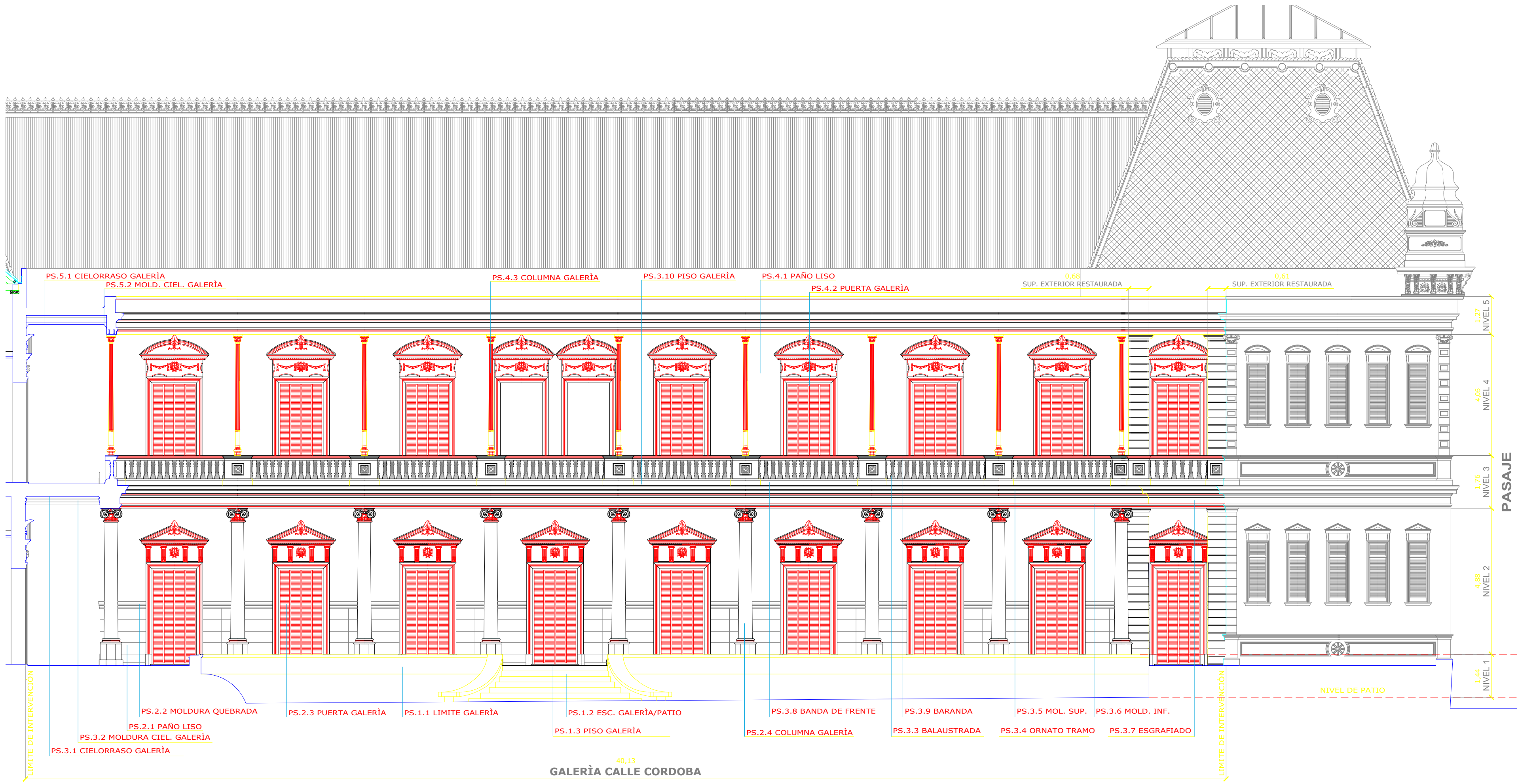
PATIO SUR - FACHADA NORTE ESC. 1:50
