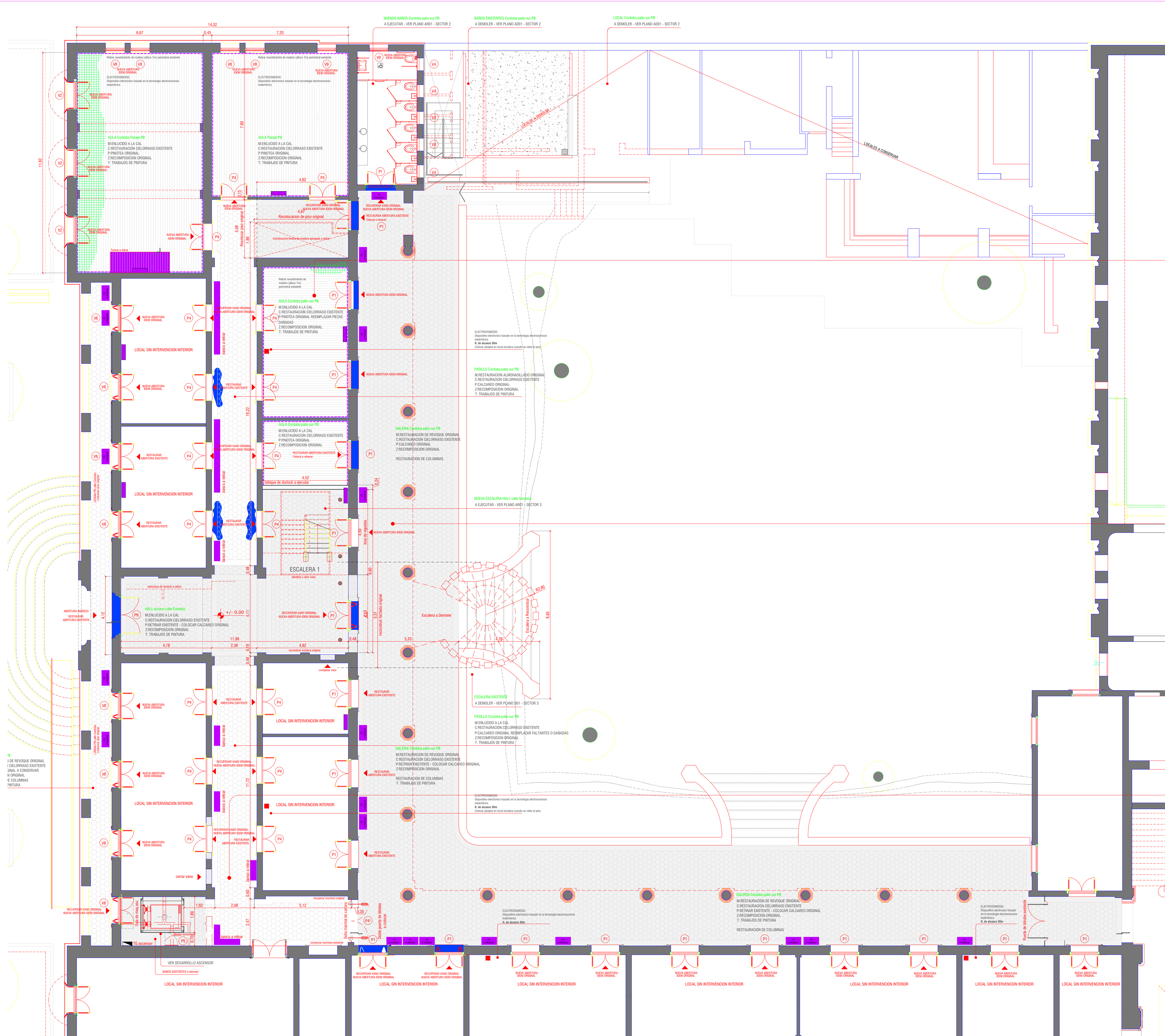
PLANTA BAJA — HALL CALLE CORDOBA ESC. 1:50
