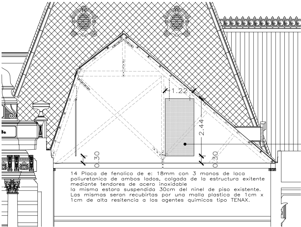
CRIA DE MURCIELAGOS SECCION TRAMO CALLE MORENO – ESC.: 1:200
