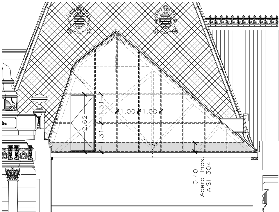
TABIQUE CORTAFUEGO SECCION TRAMO CALLE MORENO-CORDOBA – ESC.: 1:200
