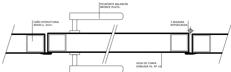
DETALLE TABIQUE CORTAFUEGO – ESC.: 1:5
