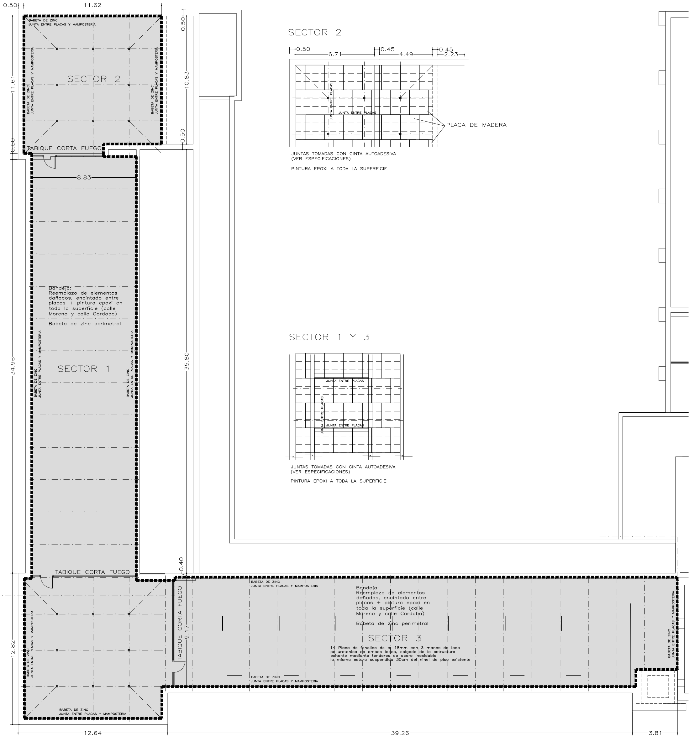
PLANTA BANDEJA SECTOR CALLE CORDOBA – ESC.: 1:200
